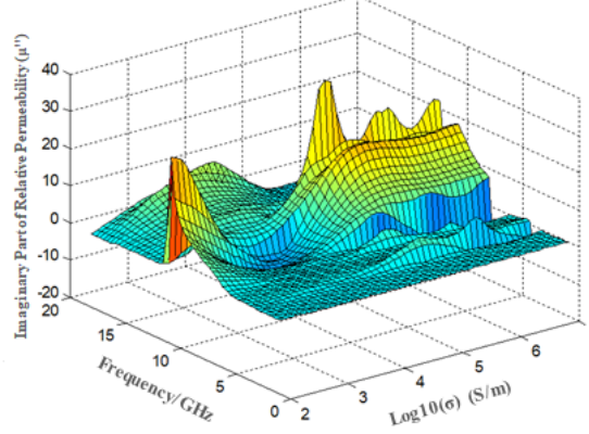
(d) Imaginary part of permeability
